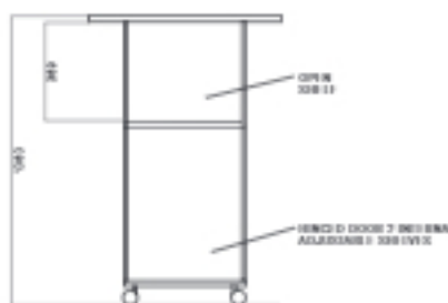
Hinged Door Option
